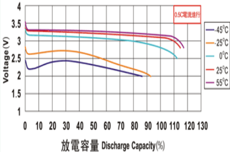
不同環境溫度下LYP類電池的放電特性曲線
