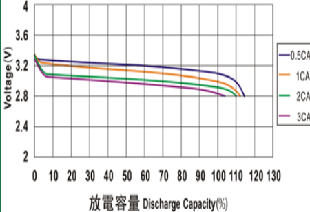
常溫下LYP類電池的放電特性曲線
