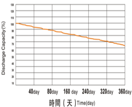
在常溫下LYP類電池的存儲特性曲線
