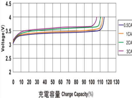
常溫下LYP類電池的充電特性曲線
