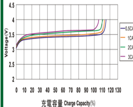
常溫下LYP類電池的充電特性曲線
