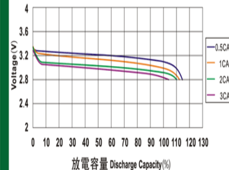
常溫下LYP類電池的放電特性曲線
