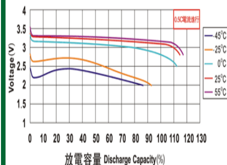
不同環境溫度下LYP類電池的放電特性曲線
