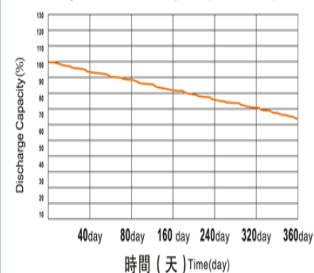
在常溫下LYP類電池的存儲特性曲線
