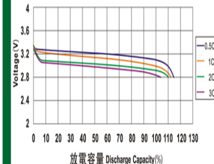
常溫下LYP類電池的放電特性曲線
