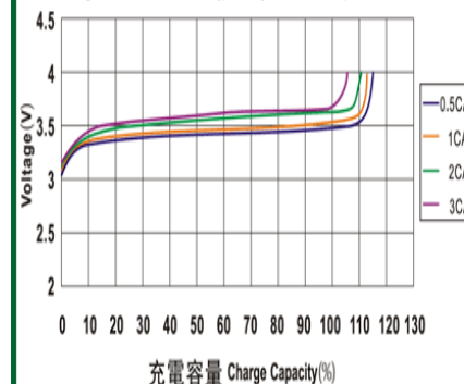
常溫下LYP類電池的充電特性曲線
