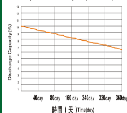
在常溫下LYP類電池的存儲特性曲線
