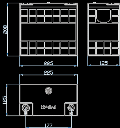
型号(MODEL): WB-LP12V40AH
