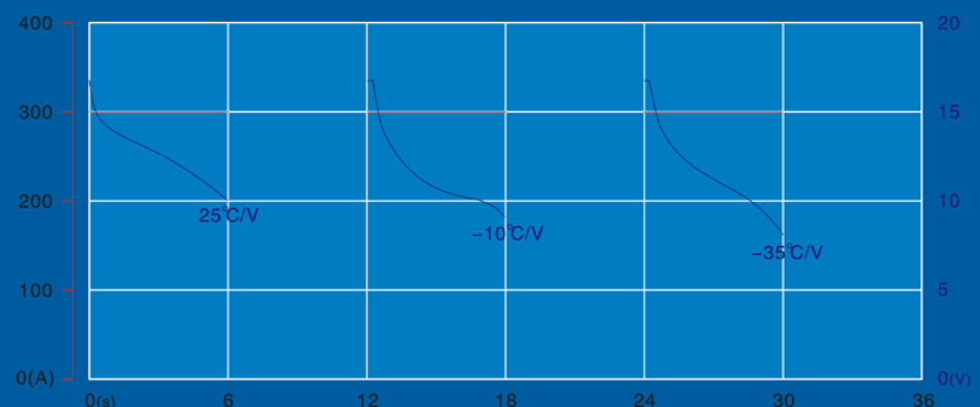
▲ WB-LP12V40AH在不同溫度環境下的脈衝放電特性 WB-LP12V40AH IMPULSE DISCHARGE AT DIFFERENT TEMPERATURE
